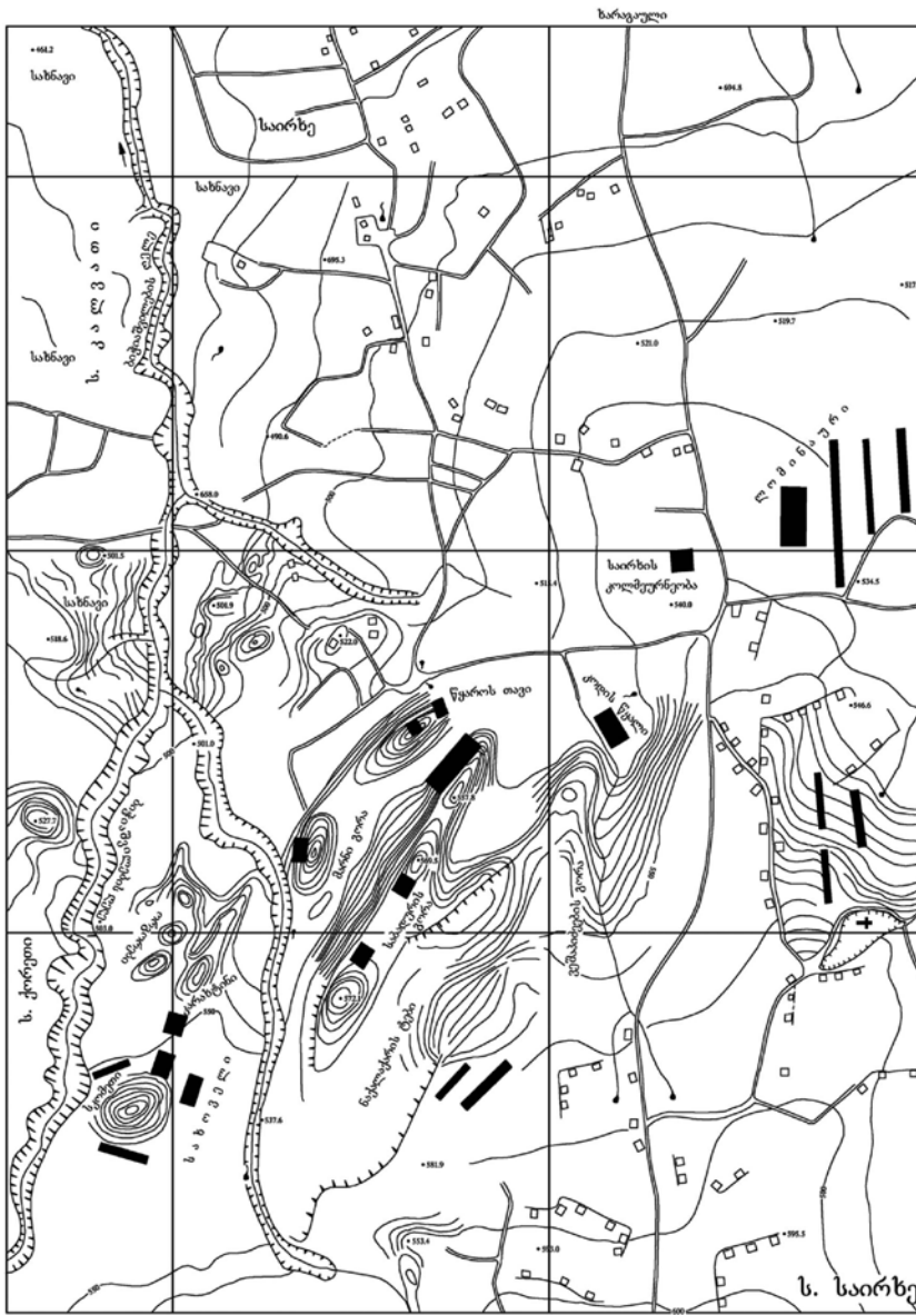
საირბის ტოპოგრაფიული გეგმა შ-ბი-1.7230
