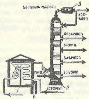
სურათი 15.12. ნავთობის უწყვეტი გა- მოხდის მილოვანი დანადგარის სქემა: 1 — მილოვანი ღუმელი; 2 — სარექტიფი- კაციო სვეტი; 3 — მაცივარი
