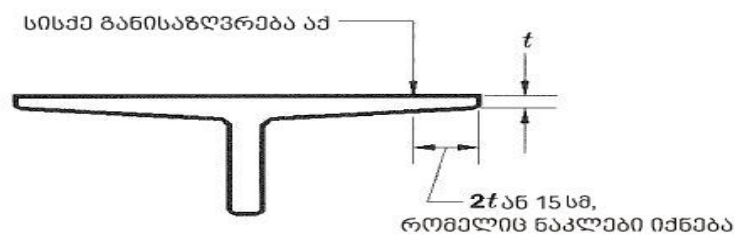
სურათი 721.2.2.1.2 ფილის სისქის განსაზღვრა დამრეცი სოფიტებისთვის
