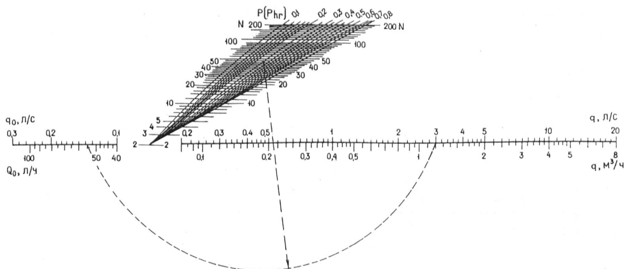
Черт.3. Номограмма для определения секундных и часовых расходов воды q при q_0 \leq 0,3 и 0,14 л/с, N \leq 200 и P > 0,1
