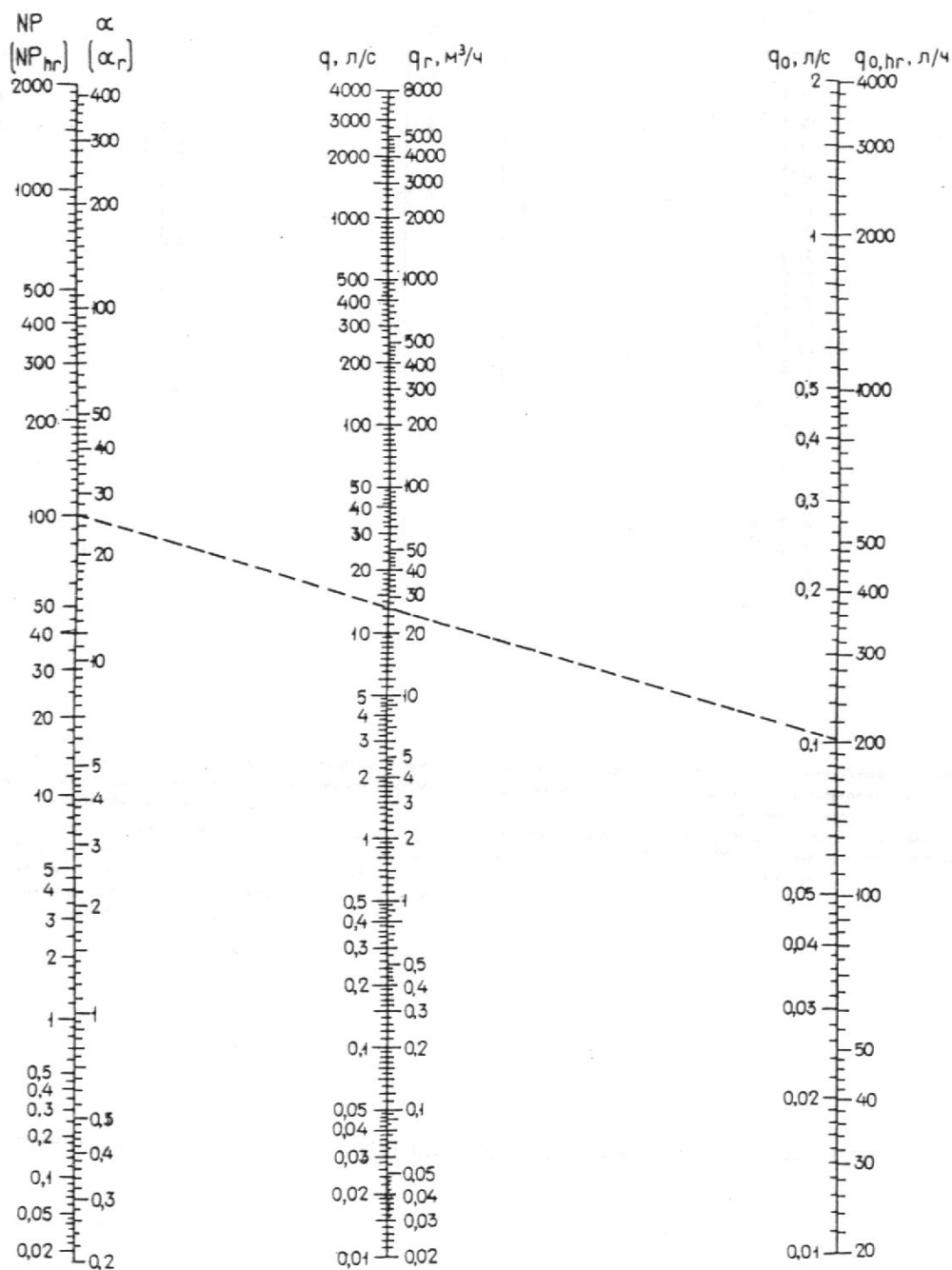
Черт.4. Номограмма для определения секундных и часовых расходов воды в зависимости от NP ( NP_{hr} ) при различных значениях q_0 , л/с, q_{0, \text{ чр}} , л/ч
