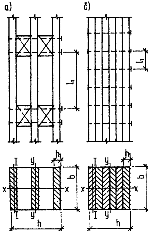
Рис. 2. Составные элементы а — с прокладками; б — без прокладок
