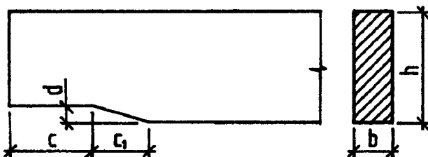
Рис. 15. Скошенная подрезка конца балки
