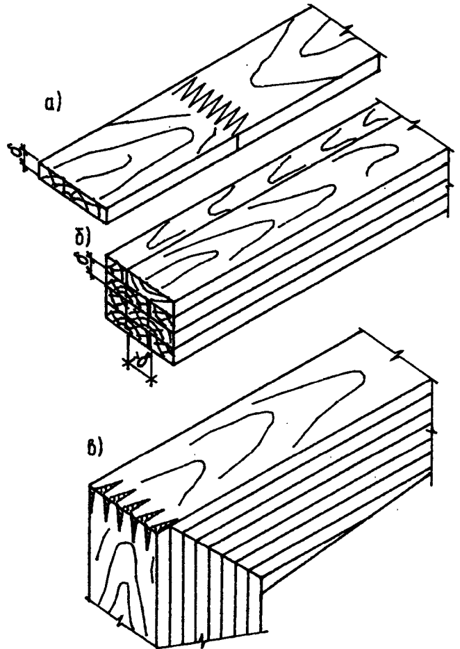
Рис. 6. Клеевые соединения
