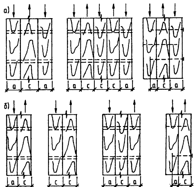
Рис. 8. Нагельные соединения а — симметричные, б — несимметричные
