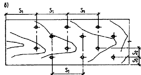
Рис. 10. Расстановка нагелей а — прямая; б — в шахматном порядке
