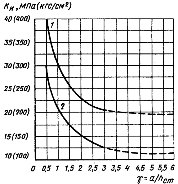
Рис. 2. Графики для определения коэффициента k_n при расположении волокон в наружных слоях фанеры вдоль пролета
