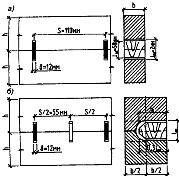
Рис. 13. Соединение на пластинчатых нагелях а — со сквозными пластинками; б — с глухими пластинками
