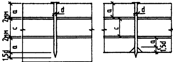
Рис. 11. Определение расчетной длины заземления конца гвоздя
