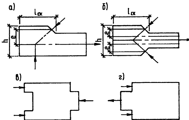
Рис. 5. Врезки в элементах соединений а — несимметричная; б — симметричная; в, г — схемы скалывания в соединениях
