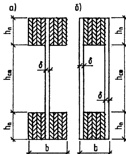
Рис. 4. Поперечные сечения клееных балок с плоской фанерной стенкой а — двутаврового сечения; б — коробчатого сечения
