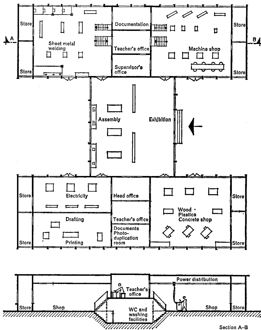
FIG. 8. Production unit.
