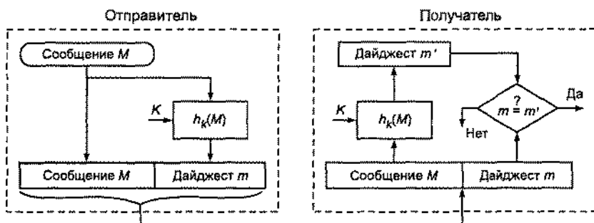
Рис. 7.3. Применение для аутентификации односторонней хэш-функции с параметром-ключом
