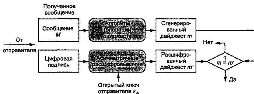
Рис. 5.7. Схема проверки электронной цифровой подписи
