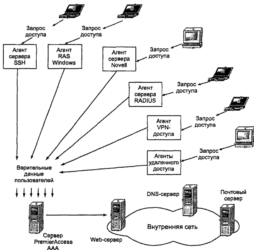
Рис. 13.2. Схема управления доступом к сети
