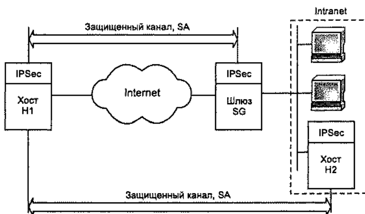
Рис. 12.10. Схема хост—шлюз, дополненная каналом хост—хост
