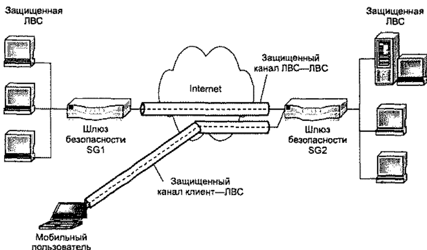
Рис. 10.4. Виртуальные защищенные каналы типа ЛВС—ЛВС и клиент—ЛВС
