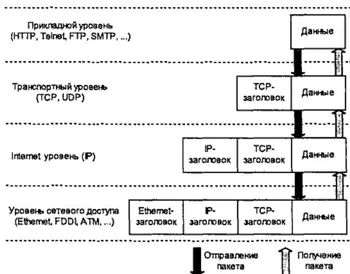
Рис. 2.3. Схема инкапсуляции данных в стеке протоколов TCP/IP
