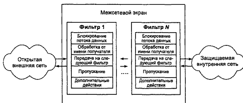
Рис. 9.2. Структура межсетевого экрана
