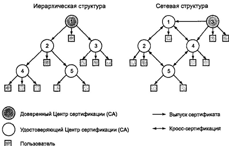
Рис. 13.10. Иерархическая и сетевая архитектуры систем управления сертификатами
