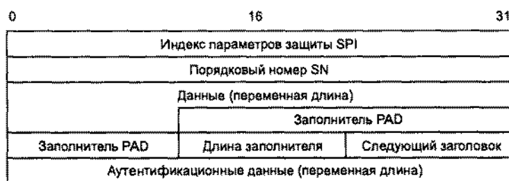
Рис. 12.5. Формат заголовка ESP
