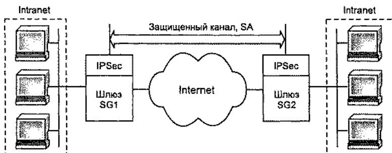
Рис. 12.9. Схема шлюз—шлюз
