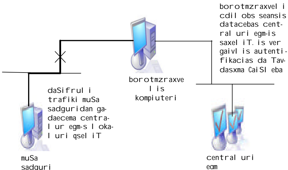
nax.1.7.2.1. daSifrva da saimedo autentifikacia SeaCerebs trafikis datacebas.
