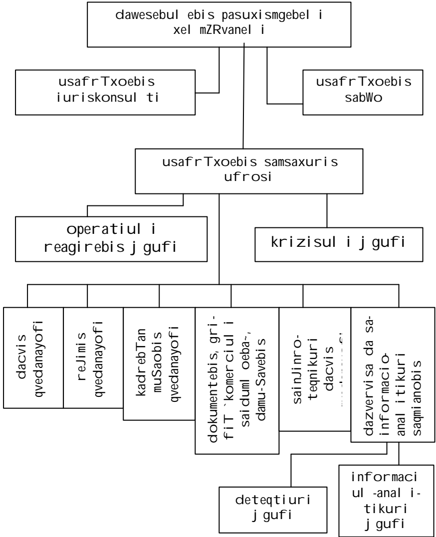
nax.1.14.3. dawesebul ebis usafrTxoebis sistemis struqturis magal iti
