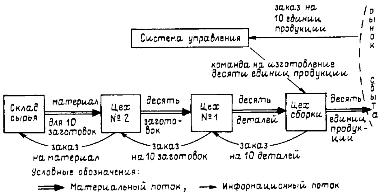
Рис. 31. Тянущая система управления материальным потоком в рамках внутрипроизводственной логистической системы
